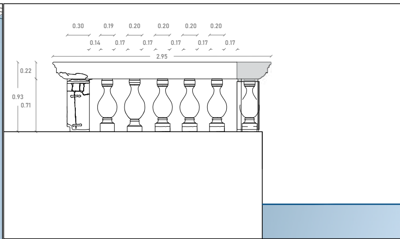
PROSPETTO SUD ANTE
