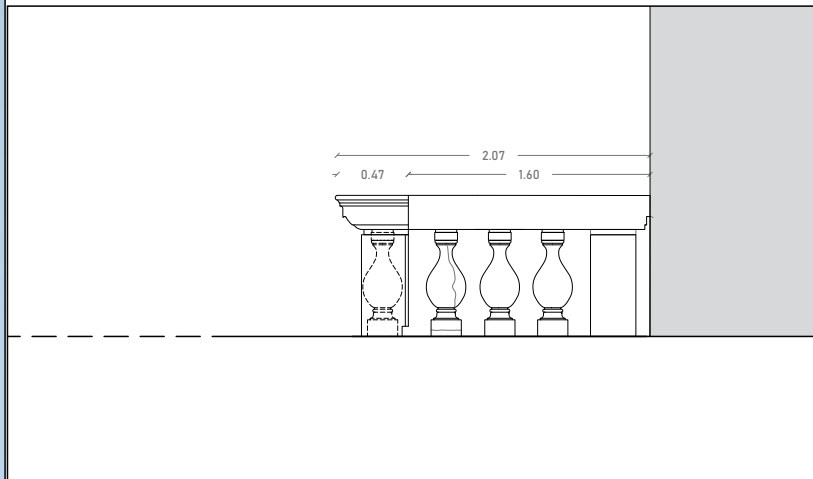
PROSPETTO EST ANTE
