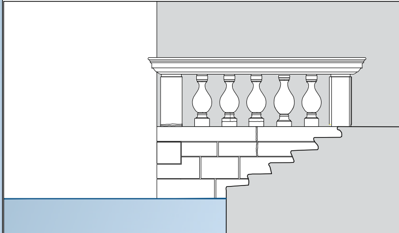
1:100 PROSPETTO OVEST ANTE
