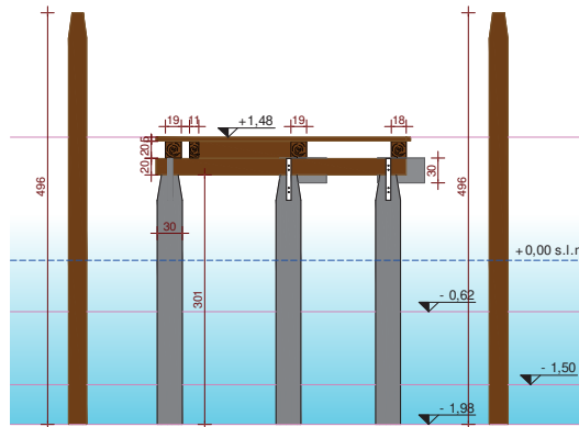
RILIEVO - PROSPETTO AA'
