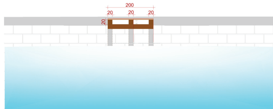
RILIEVO - PROSPETTO AA'
