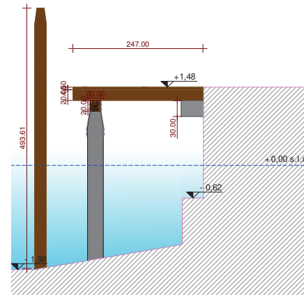
RILIEVO - PROSPETTO BB'
