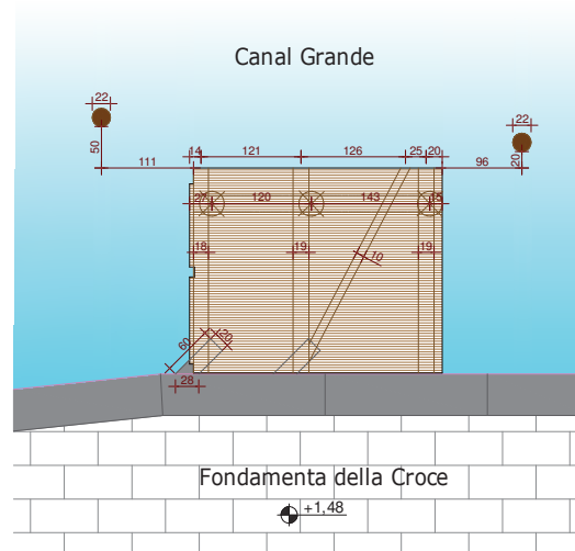
DETTAGLIO STRUTTURA LIGNEA IN PIANTA
