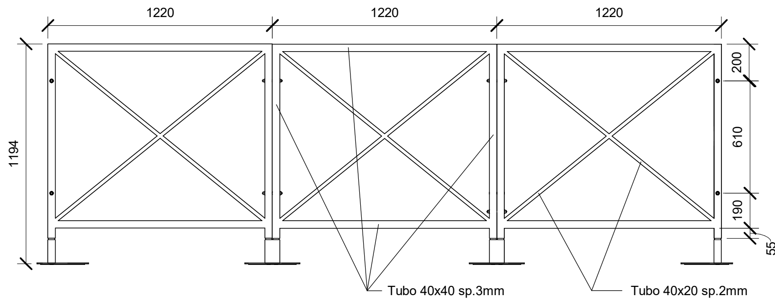
1 Lato opposto al cancello 1 : 20
