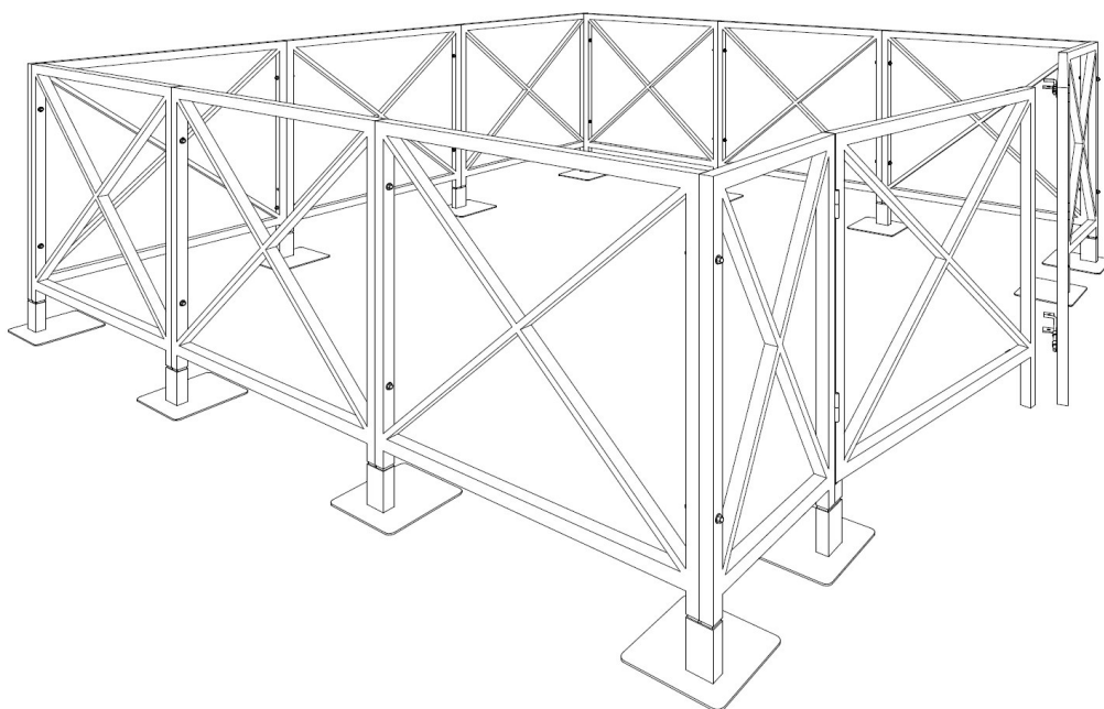
Figura 4-6 Schema generale della recinzione tipo
