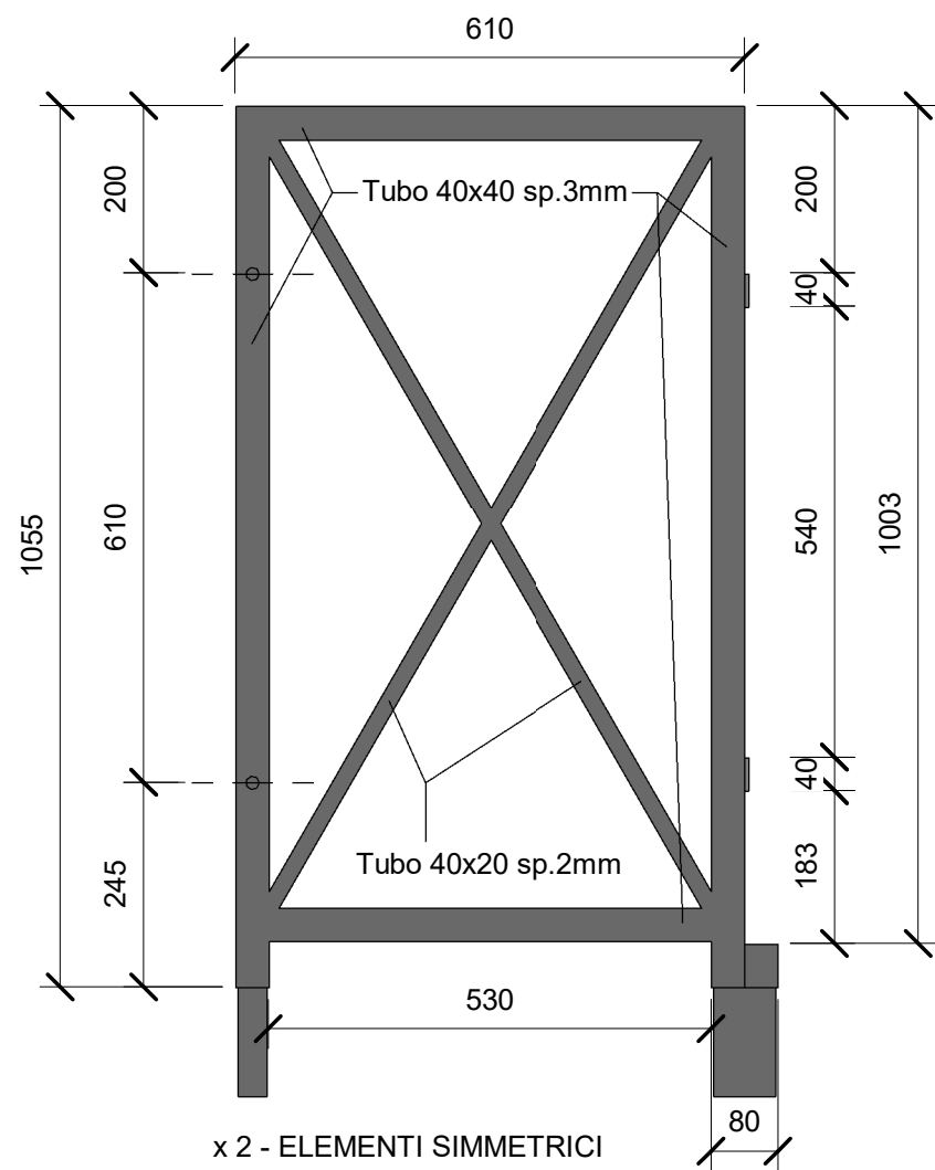
2 Spalletta cancello 1 : 10
