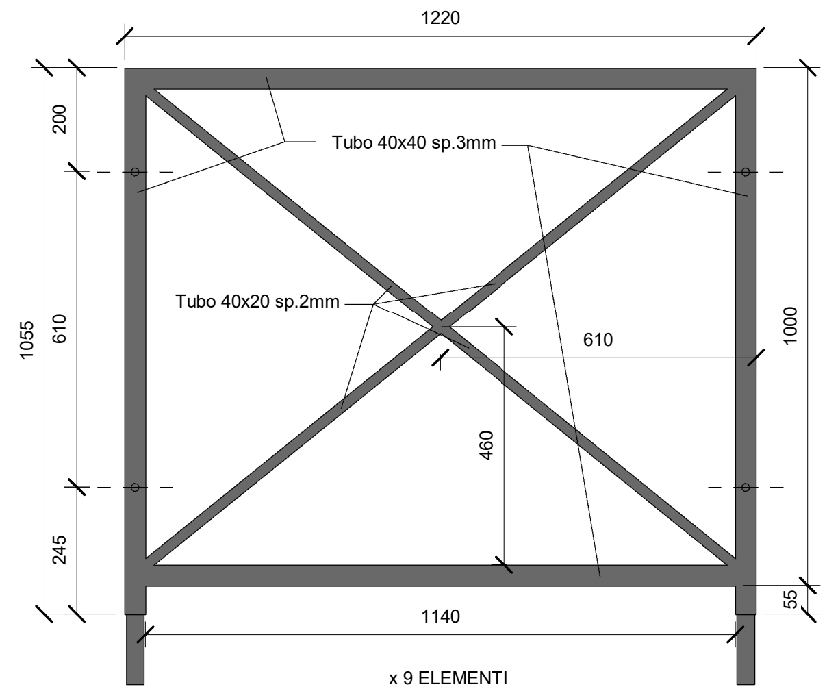
5 Pannello tipo 1 : 10
