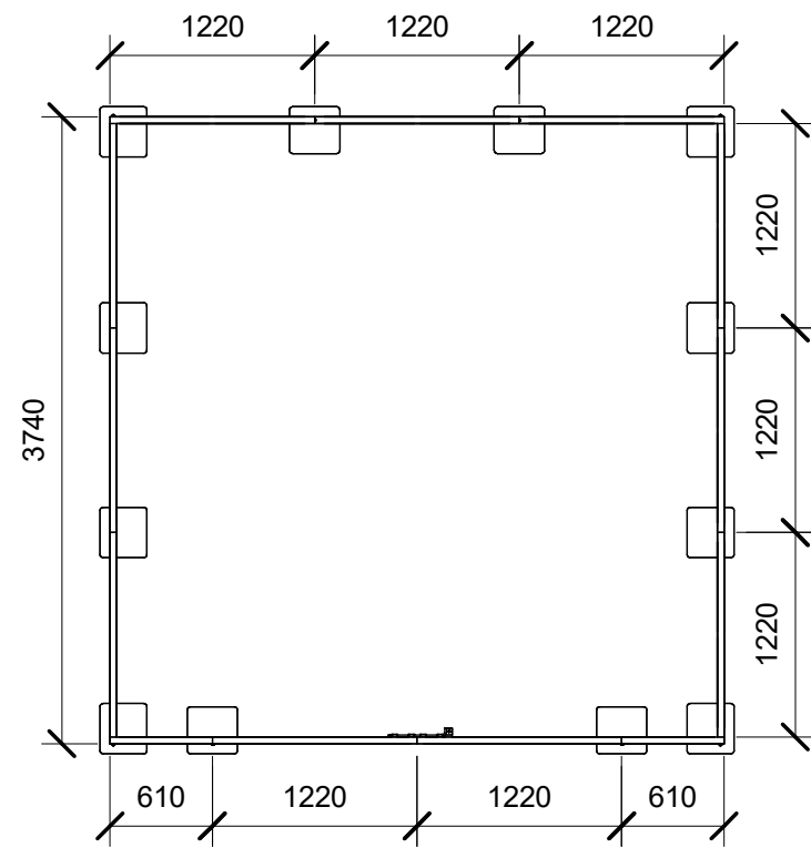
1 Planimetria recinto 1 : 50
