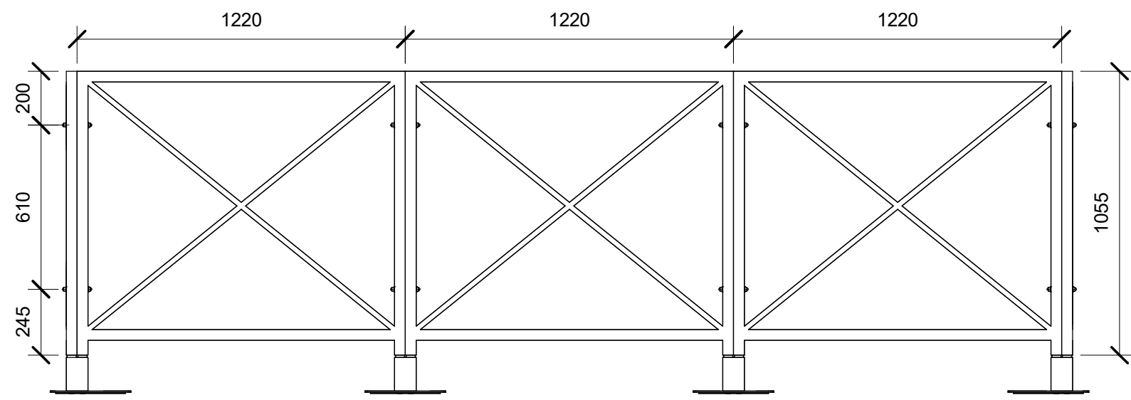
2 Vista laterale 1 : 20
