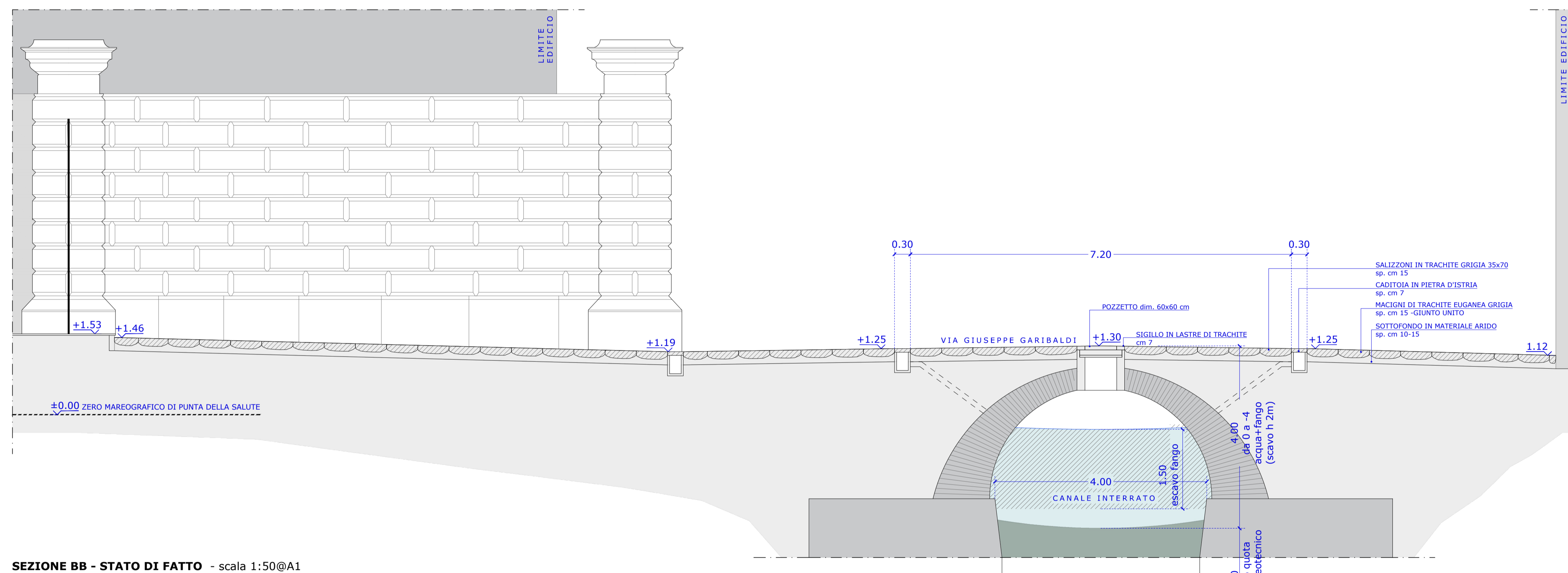
SEZIONE BB - STATO DI FATTO - scala 1:50@A1
