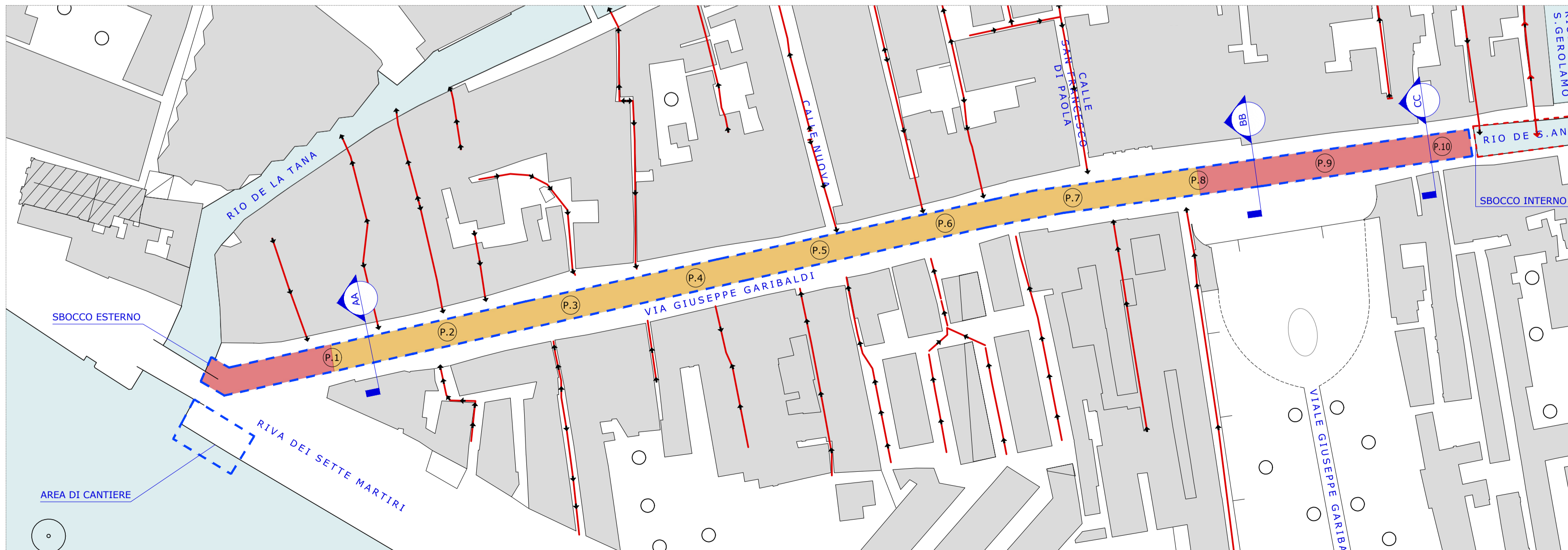
PLANIMETRIA DI INQUADRAMENTO - RIO TERA' GARIBALDI - scala 1:1000@A1
