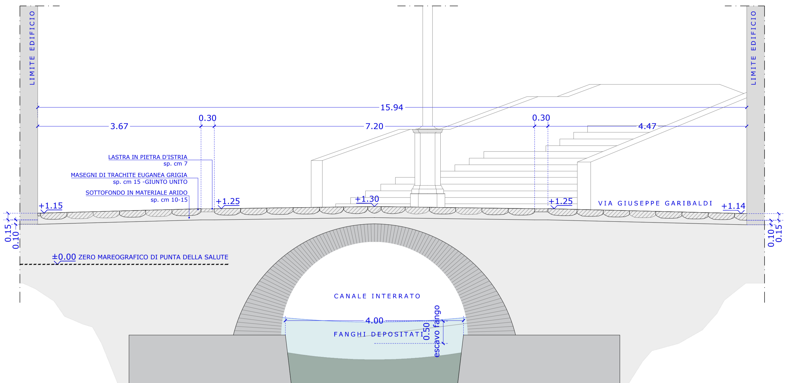
SEZIONE AA - scala 1:50@A1
