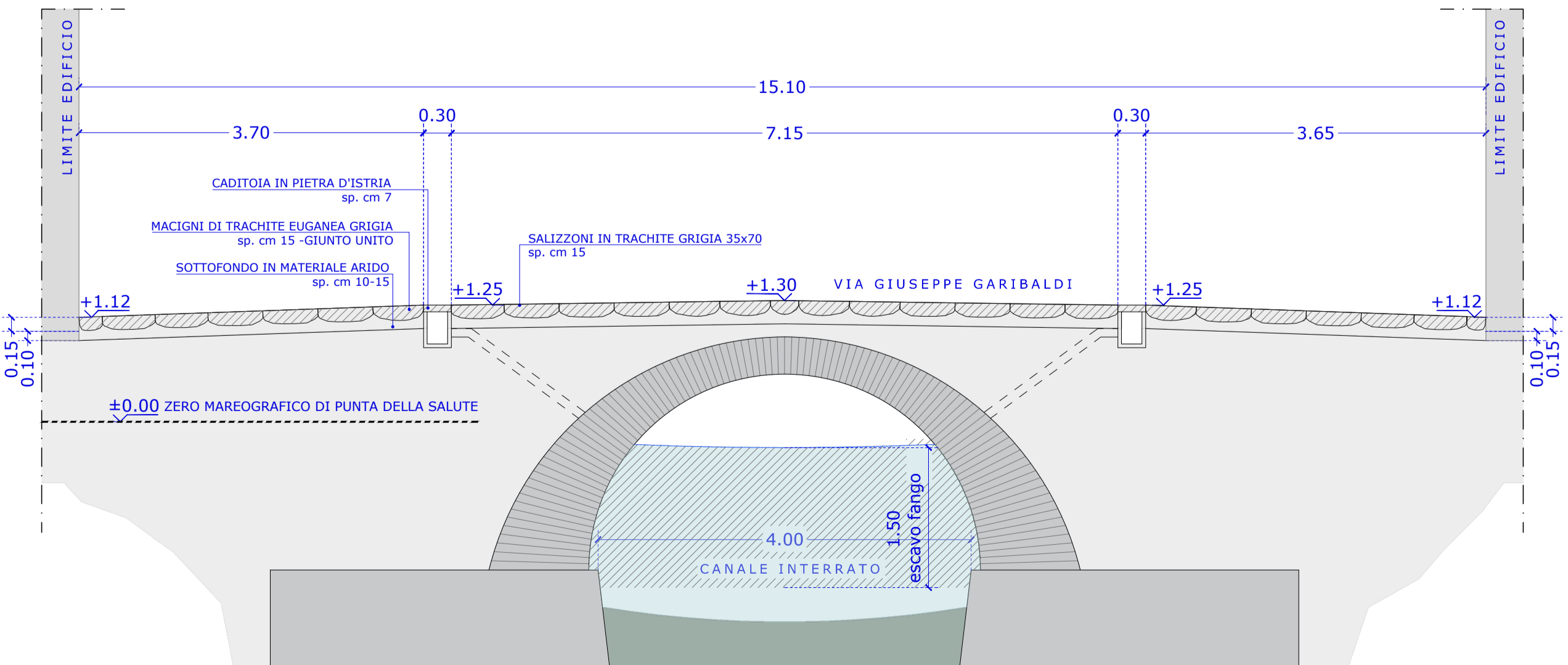
SEZIONE CC - STATO DI FATTO - scala 1:50@A1
