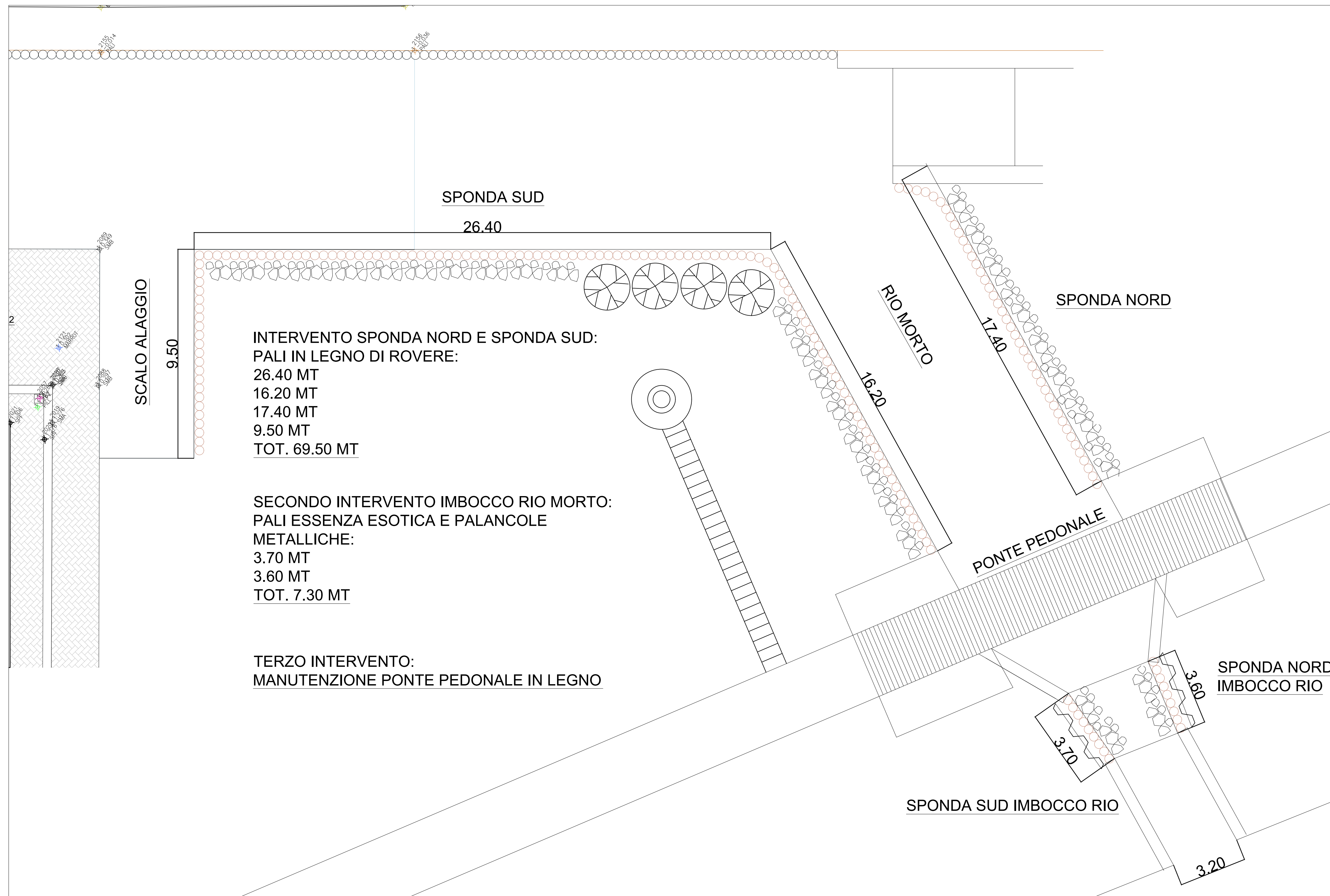
Progetto _ Planimetria - scala 1:200
