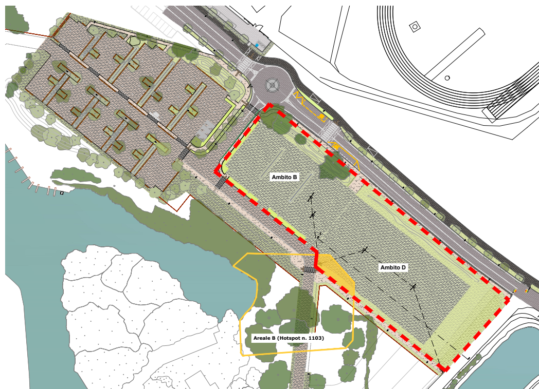
Planimetria Stato di Fatto con indicazione dell'area interessata dal progetto di bonifica Areale B (Hotspot n. 1103)
