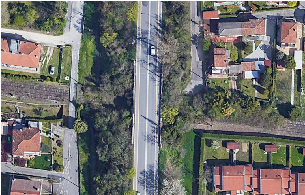
Fig. 1 – Foto aerea del tratto centrale del cavalcaferrovia
