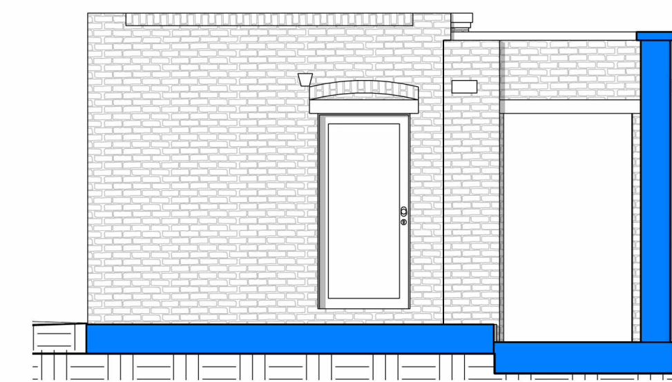
PROSPETTO NORD STATO DI PROGETTO Scala 1 : 50 | STATO DI PROGETTO
