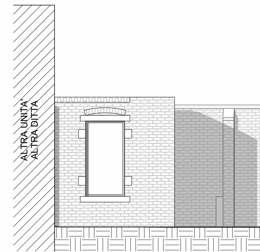
PROSPETTO EST - STATO DI PROGETTO Scala 1 : 50 | STATO DI PROGETTO
