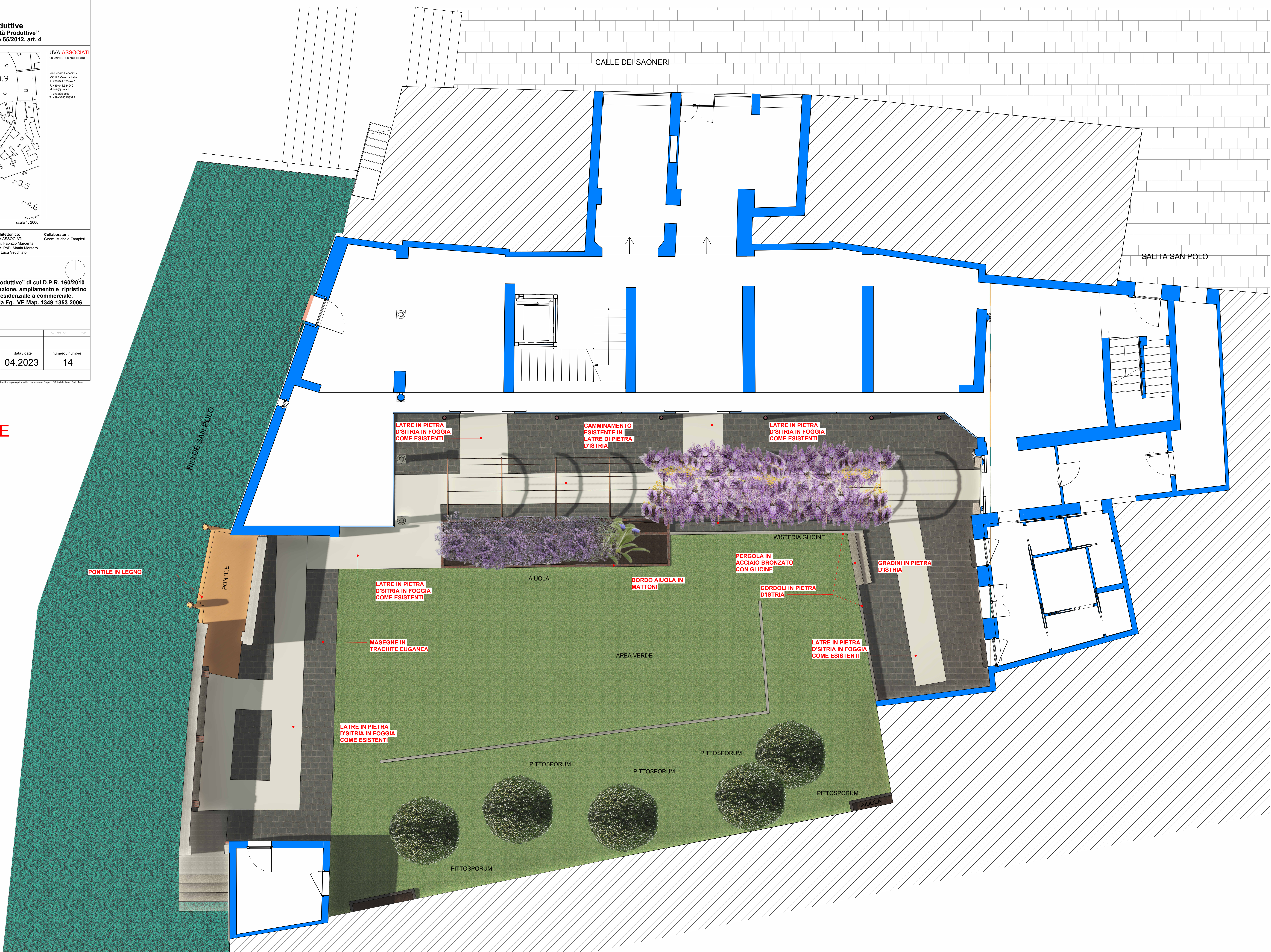
PLANIMETRIA SISTEMAZIONE ESTERNA Scala 1:50 | STATO DI PROGETTO
