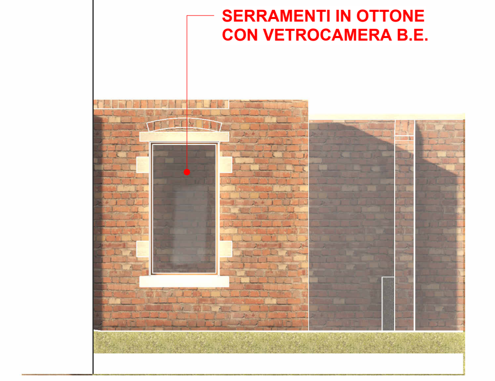
PARTICOLARE PROSPETTICO EST Scala: 1:50 | STATO DI PROGETTO
