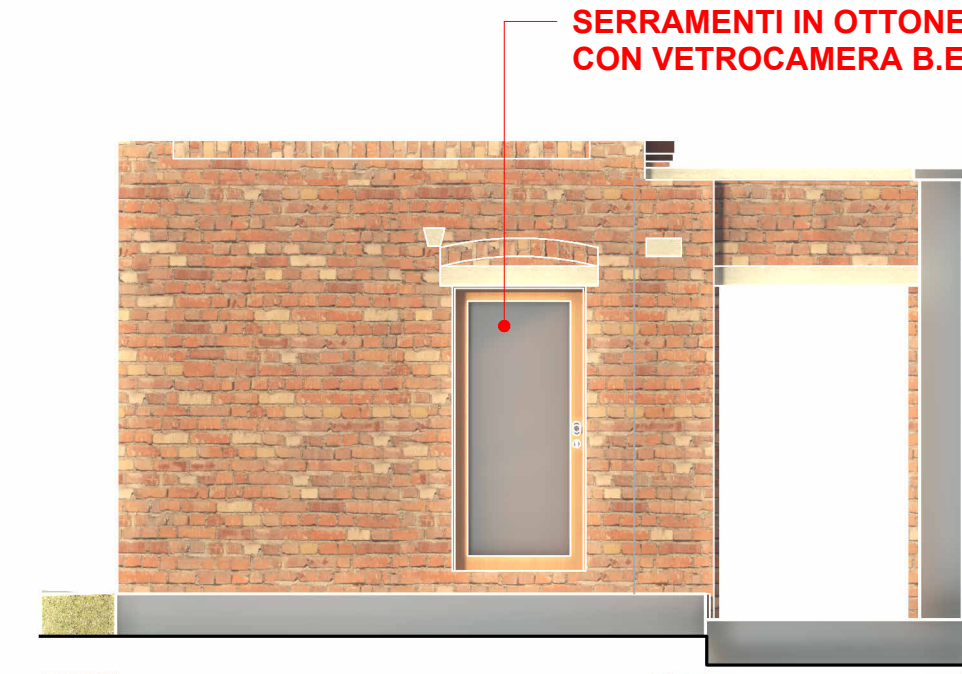
PARTICOLARE PROSPETTICO NORD Scala: 1:50 | STATO DI PROGETTO
