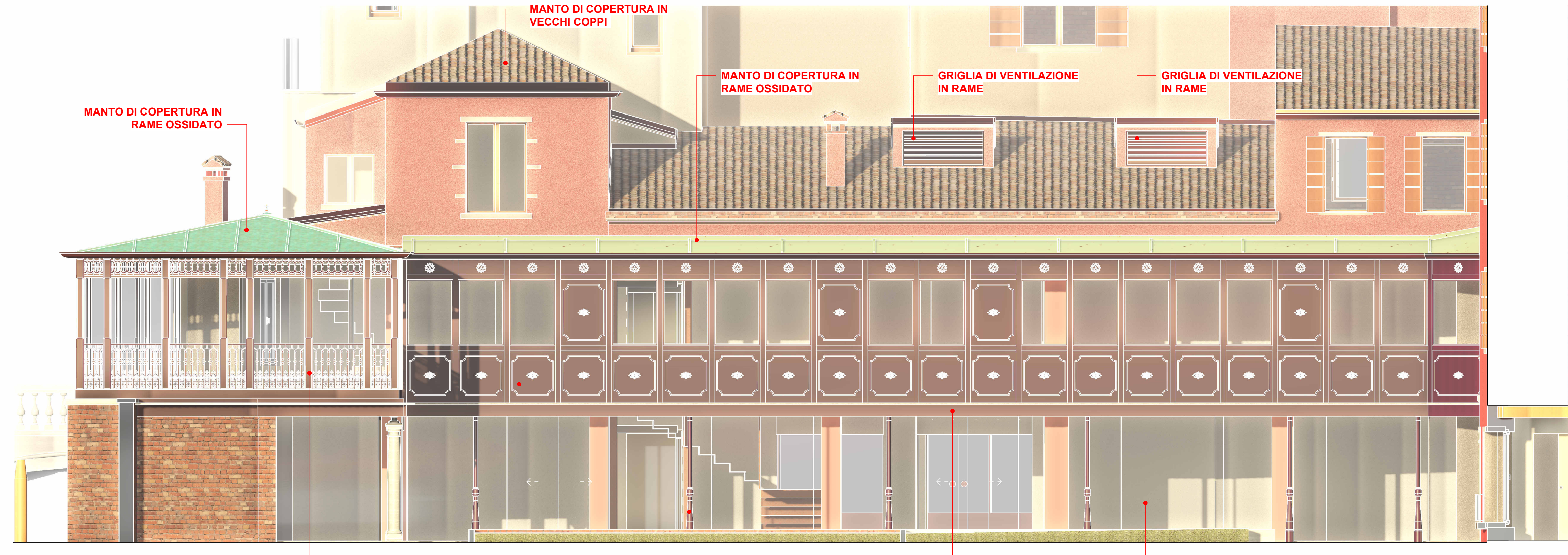
PARTICOLARE PROSPETTICO SUD Scala: 1:50 | STATO DI PROGETTO
