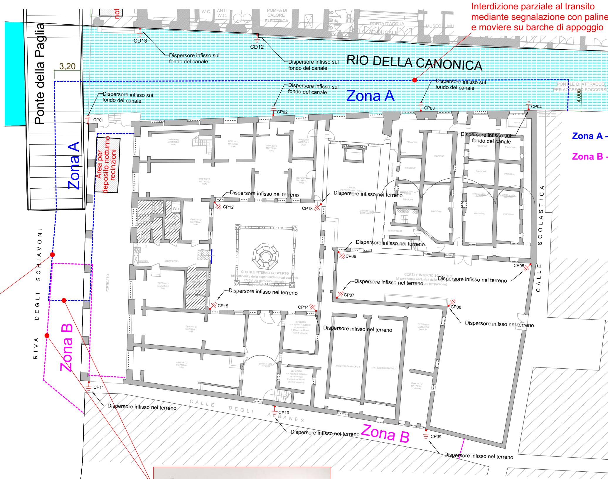
Recinzione mobile di cantiere altezza 2 mt. Posizionata alle ore 7:00 e rimossa alle ore 18.00 per intercludere il transito pedonale durante le lavorazioni su fune sulla copertura e sulle facciate di Palazzo Prigioni Nuove
