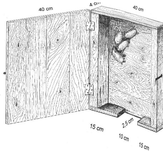
Casetta-rifugio per pipistrelli — disegno tratto da "Pipistrelli" AA.VV. (2003), Ente Gestore Parchi ... del lago Maggiore
