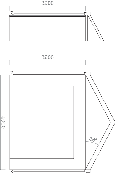
SEZ A-A
