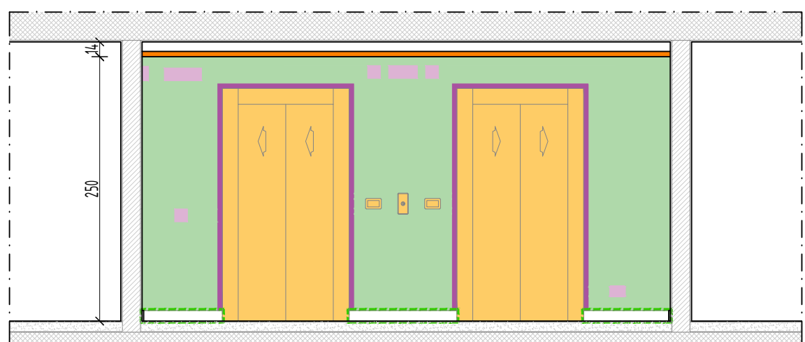
PROSPETTO PIANO TERRA - 1:50
