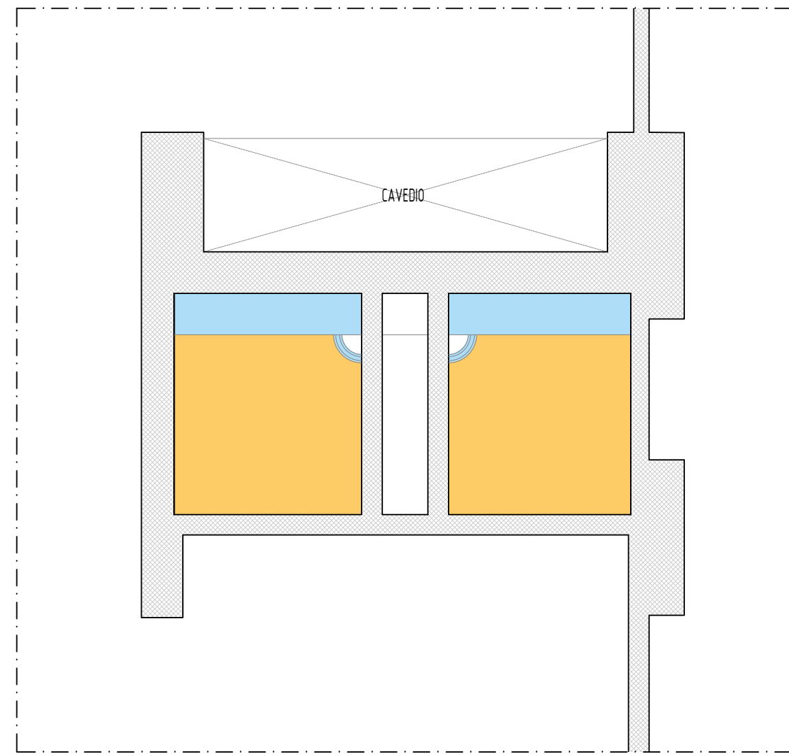
FOSSA ASCENSORI - 1:50
