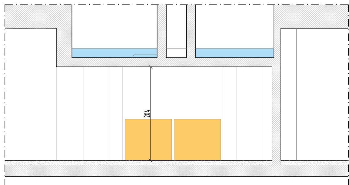
PROSPETTO PIANO INTERRATO - 1:50
