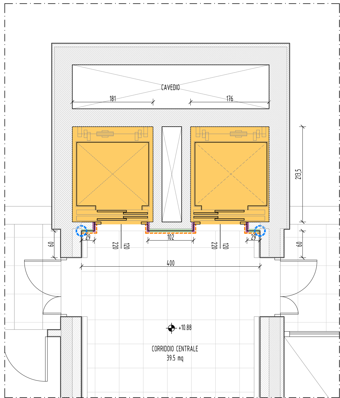
PIANO TERZO - 1:50
