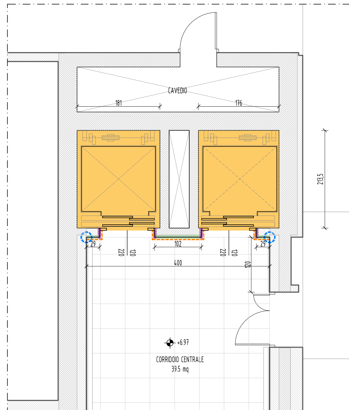
PIANO SECONDO - 1:50
