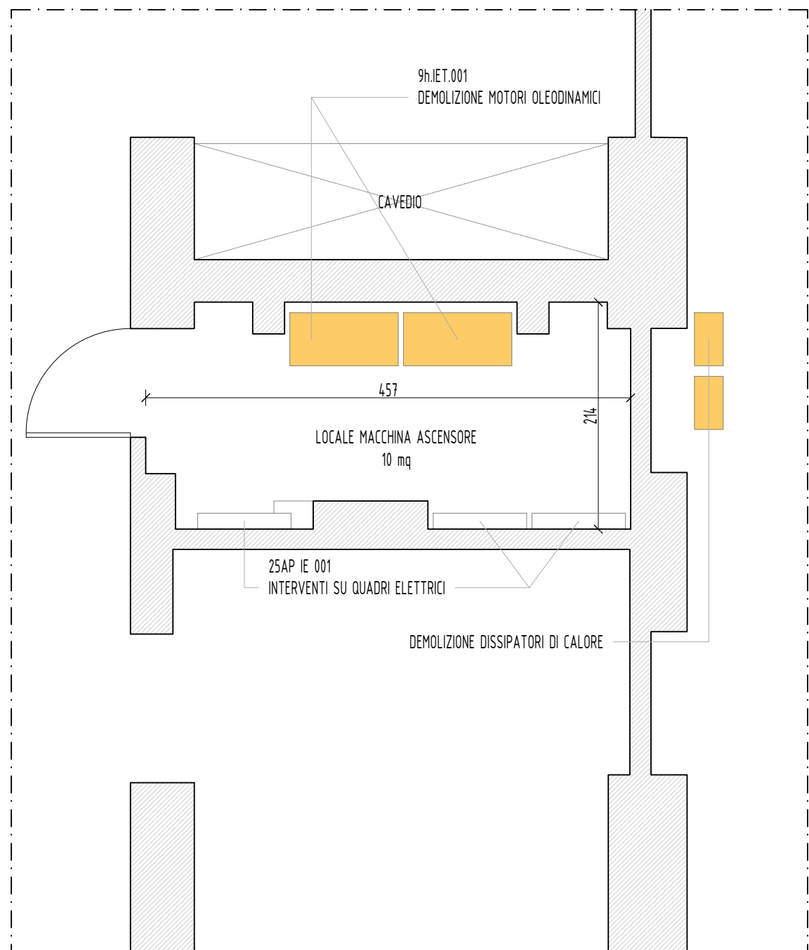
PRIMO PIANO INTERRATO - 1:50
