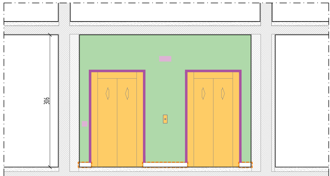
PROSPETTO PIANO QUARTO - 1:50
