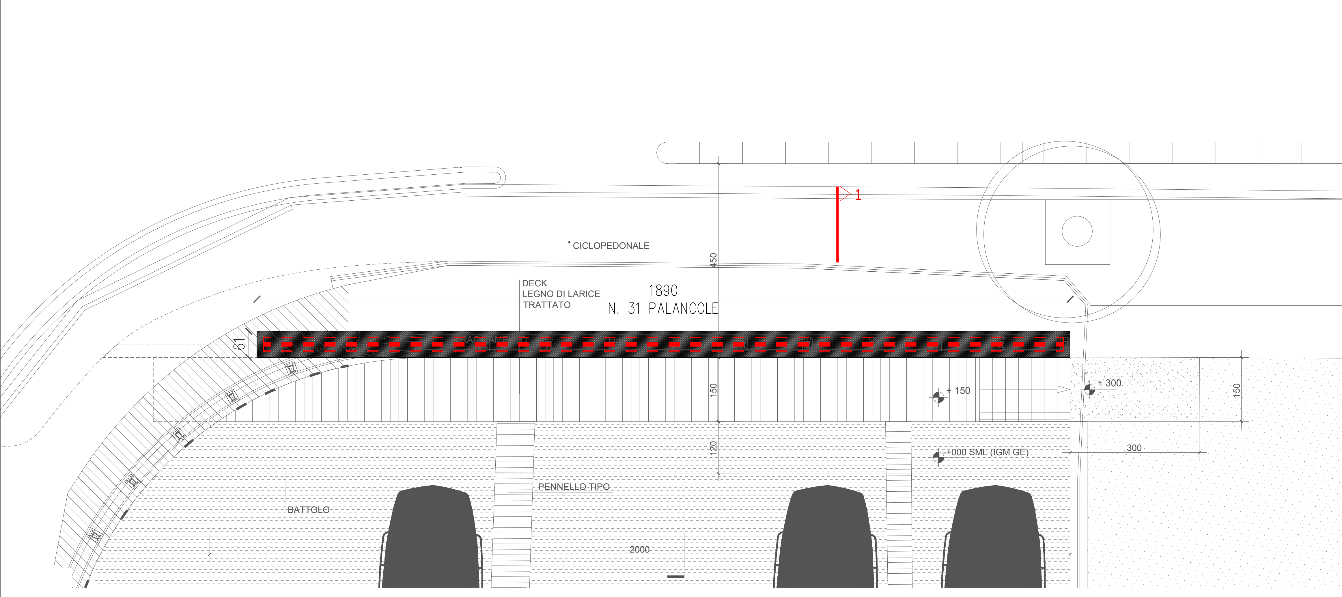
01. PLANIMETRIA PALANCOLATO INTERVENTO 2_scala 1:50
