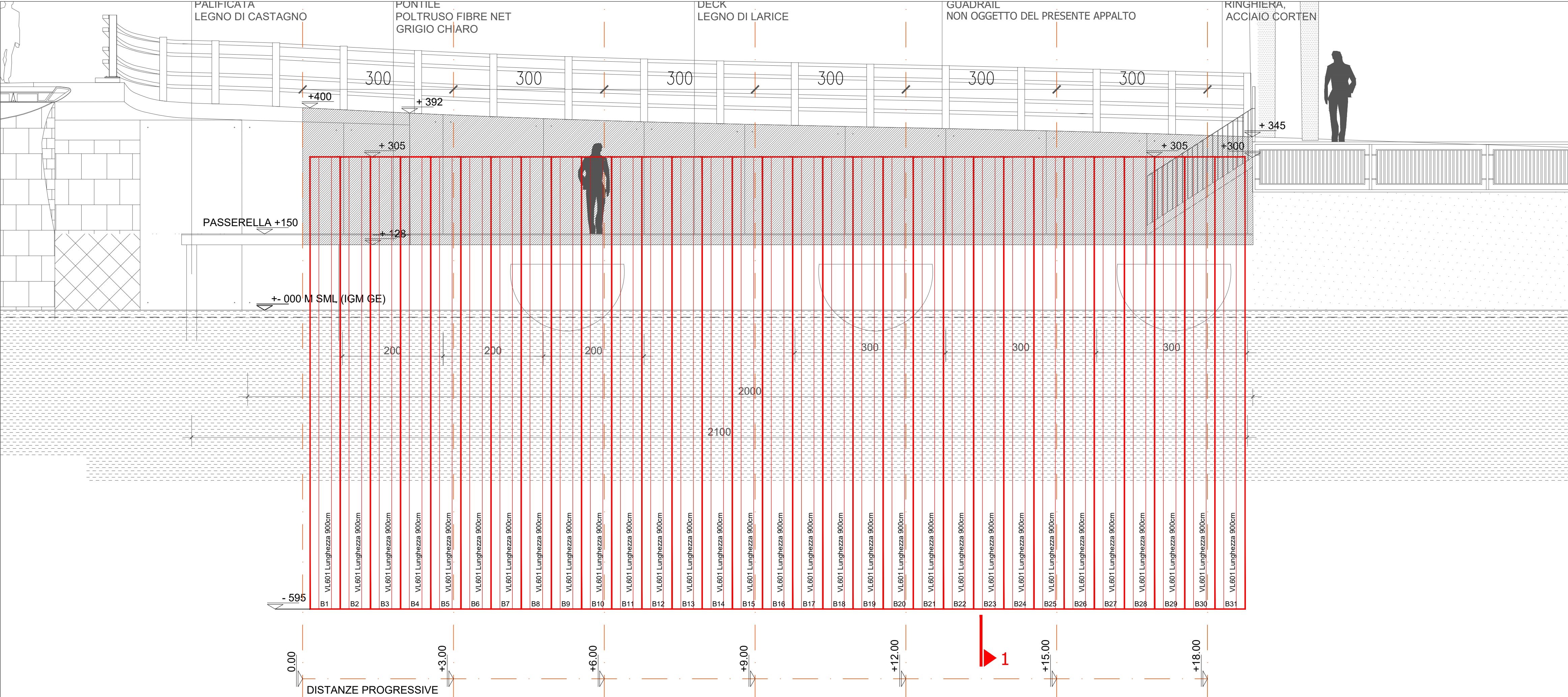
02. PROSPETTO PALANCOLATO INTERVENTO 2_scala 1:50
