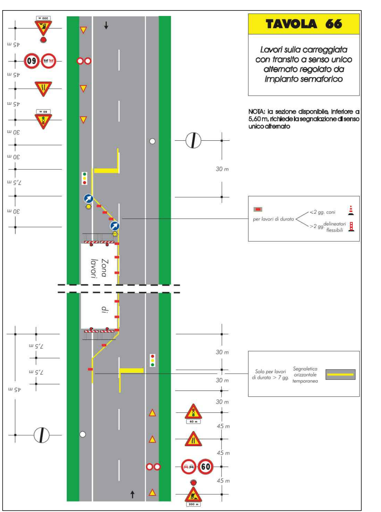
SCHEMA TIPO SEGNALETICA
