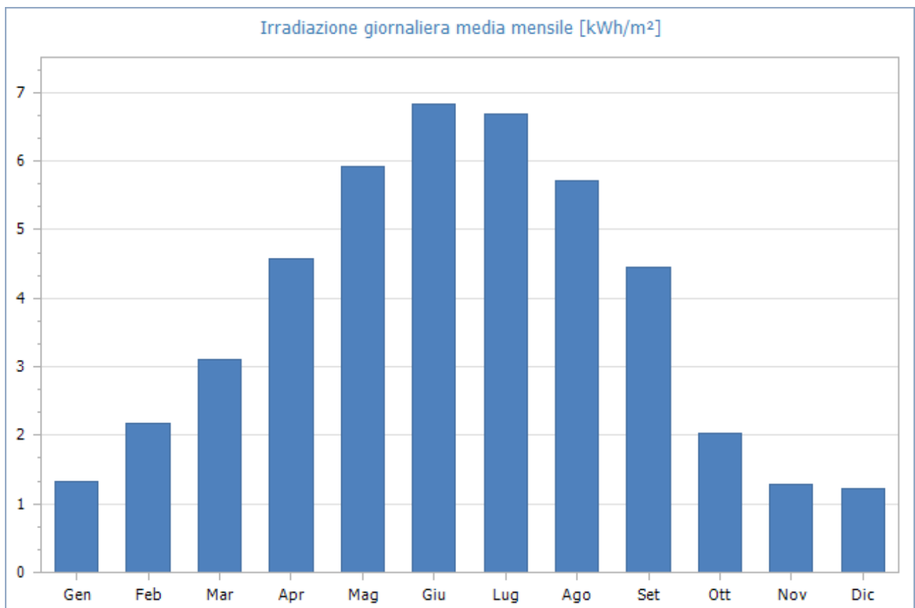
Fig. 1: Irradiazione giornaliera media mensile sul piano orizzontale [kWh/m 2 ]- Fonte dati: UNI 10349:2016 - Stazione di rilevazione: Campagna Lupia - Valle Averso
