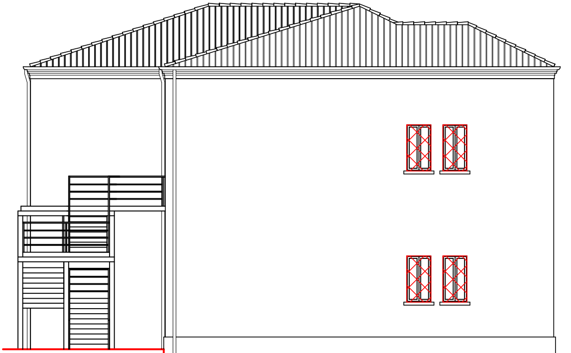
PROSPETTO EST - Lato canale
