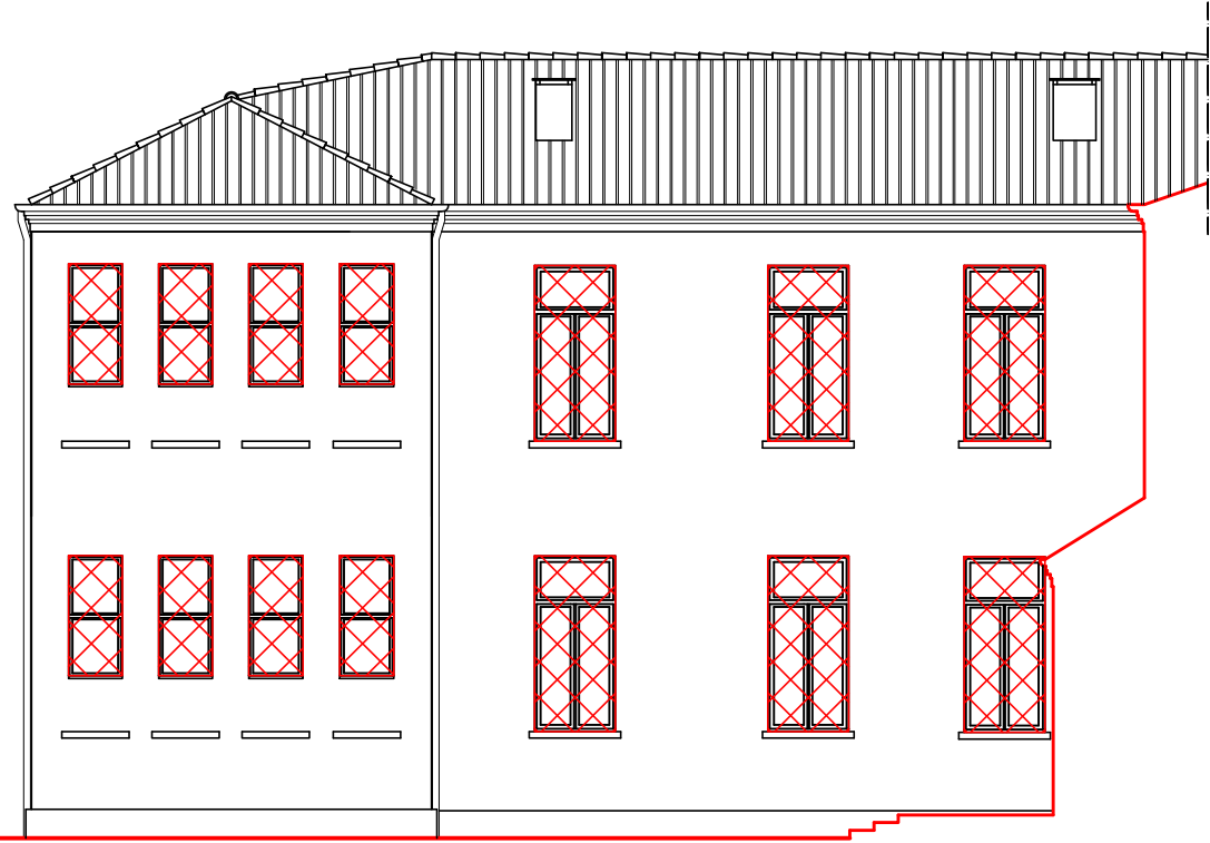
PROSPETTO NORD - Lato Corte
