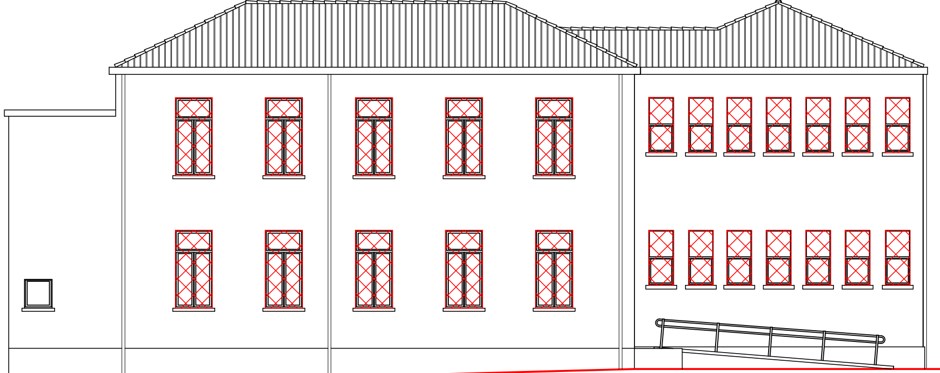
PROSPETTO NORD - Lato Campiello San Vito
