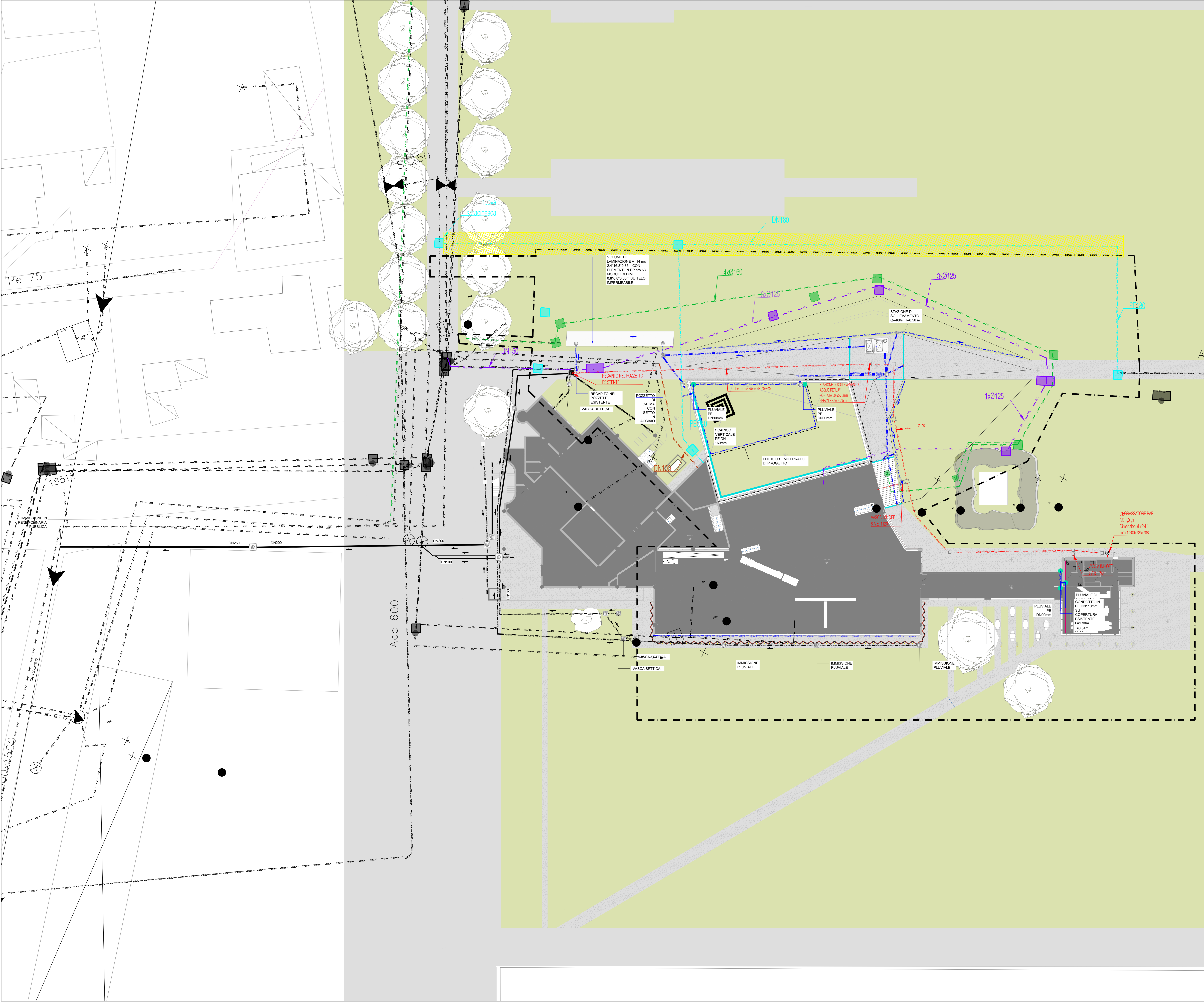
01 Planimetria stato di progetto 1:200
