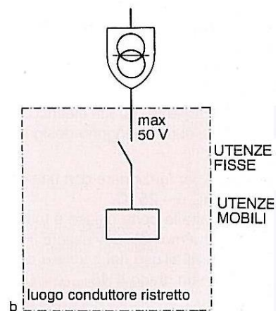
Figura 7 - schema alimentazione luogo conduttore ristretto
