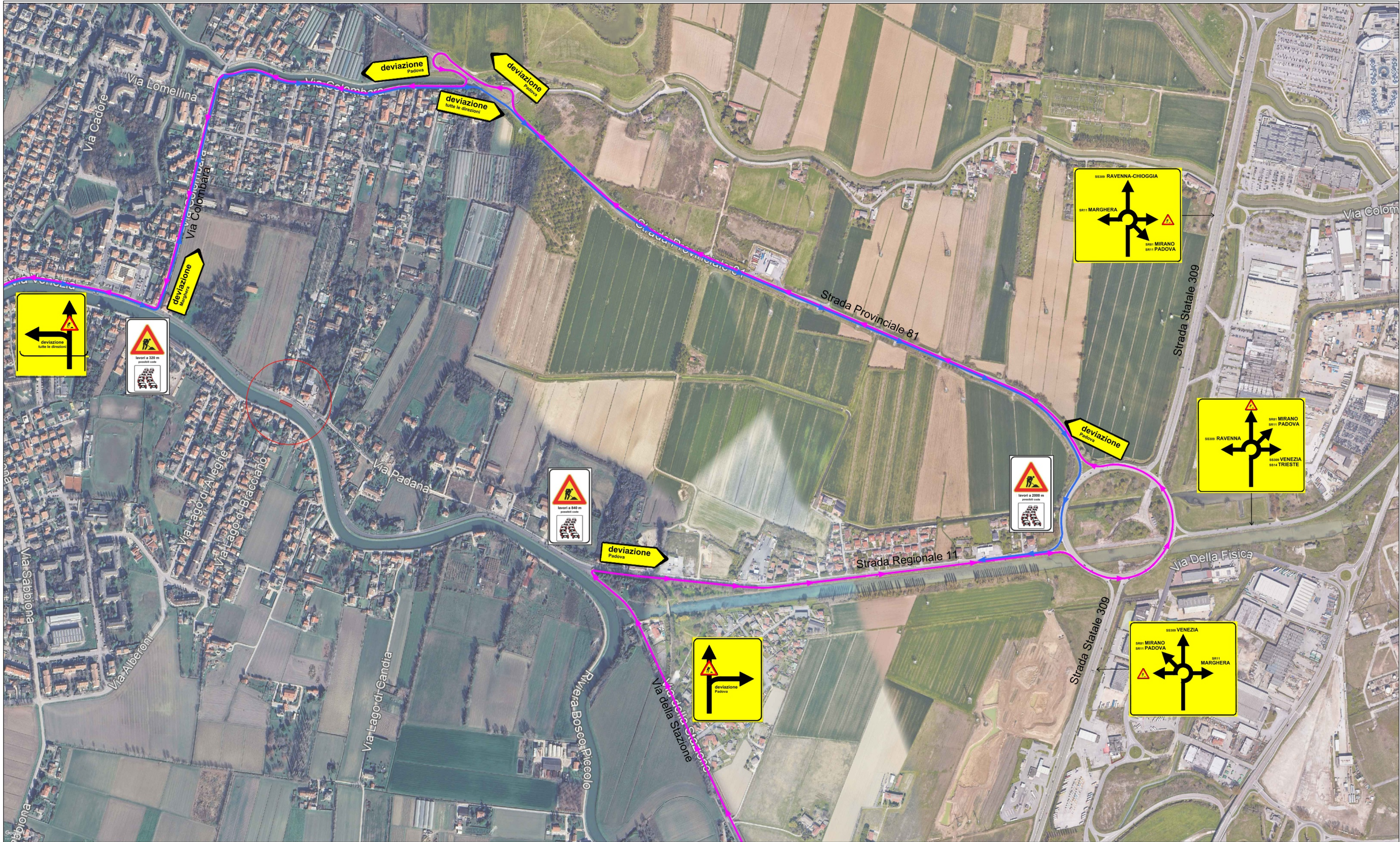
PLANIMETRIA DEVIAZIONI VIABILITÀ CANTIERE
