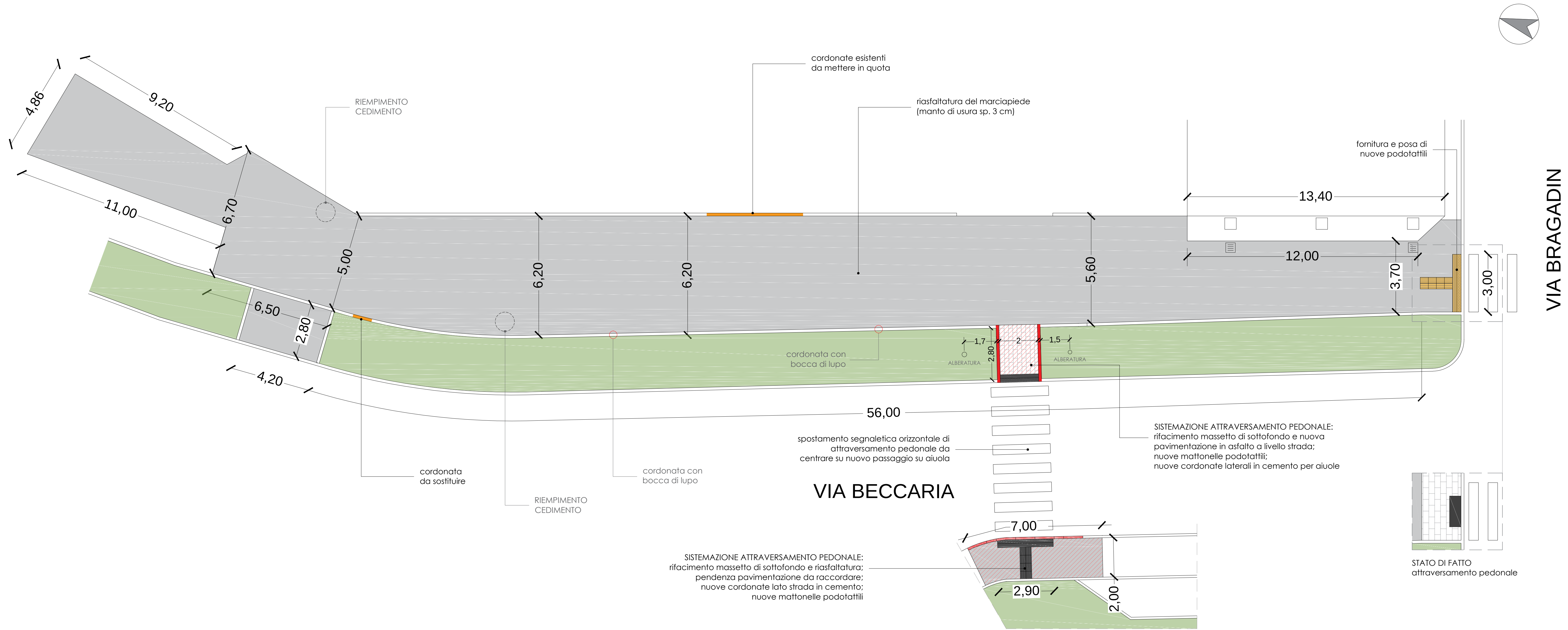
STATO DI PROGETTO - SCALA 1:100
