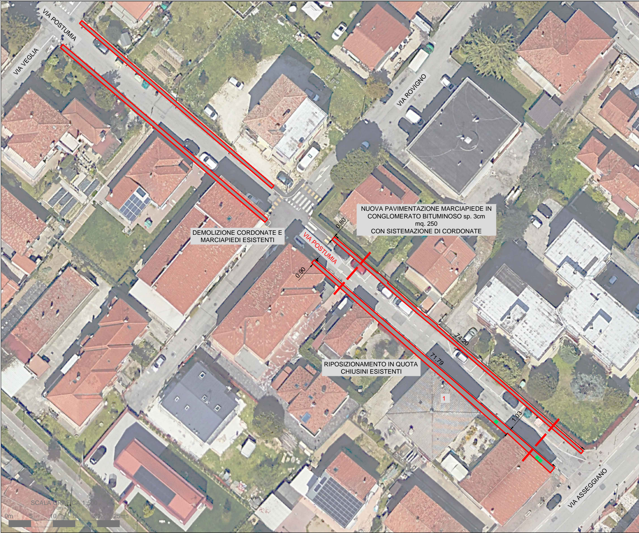
A - INTERVENTO DI FRESATURA E RIFACIMENTO MANTO IN CONGLOMERATO BITUMINOSO - sp. 3 cm
