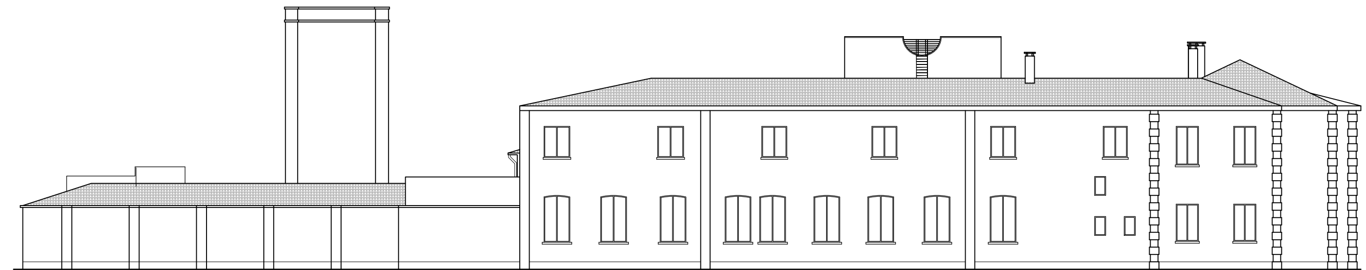
PROSPETTO NORD Scala 1:200
