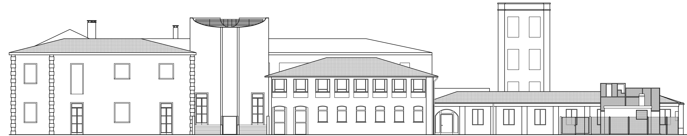
PROSPETTO SUD Scala 1:200
