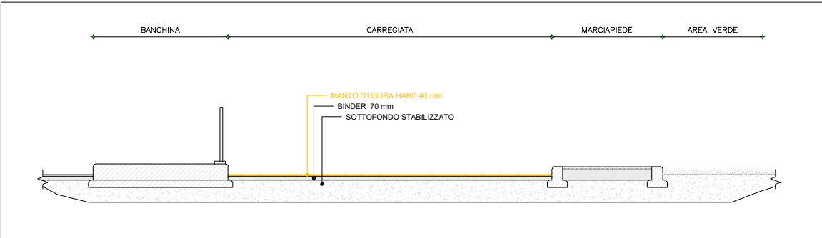
Rifacimento di solo strato di usura con fresatura e posa tappeto Hard sp. 4cm
