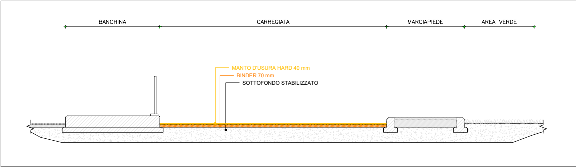
Bonifica e rifacimento strato di usura con fresatura e posa di Binder sp. 7cm e tappeto Hard sp. 4cm
