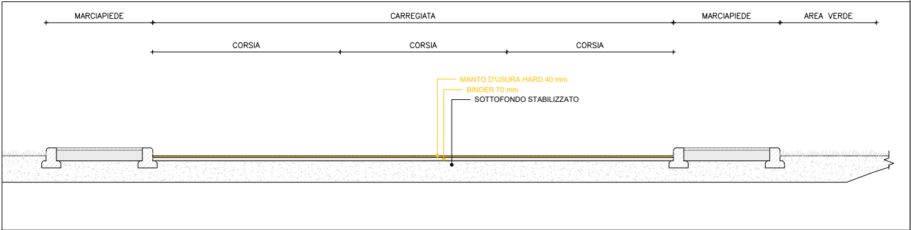
Fase A_Rifacimento di solo strato di usura con fresatura e posa tappeto Hard sp. 4cm
