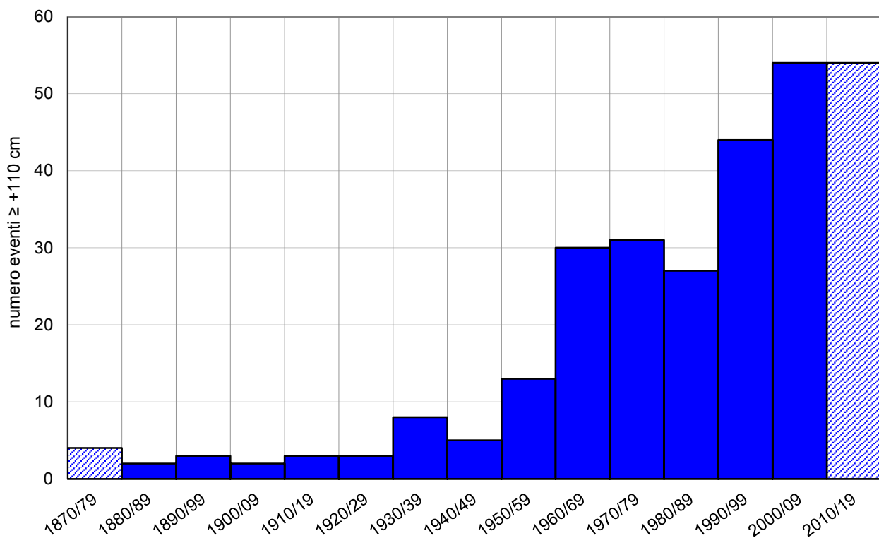
Figura 6 - Distribuzione decennale delle maree \geq +110 cm registrate a Venezia dal 1872 al 2015 Un colore diverso evidenzia il decennio incompleto
