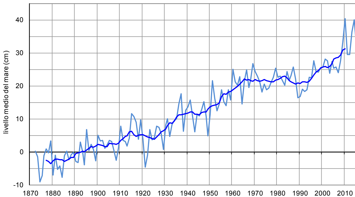
Figura 1 - Livello medio del mare a Venezia dal 1872 al 2015 e media mobile su 11 anni
