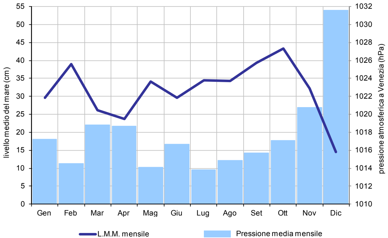
Figura 3 - Variazione del livello medio mare e della pressione media mensili nel 2015
