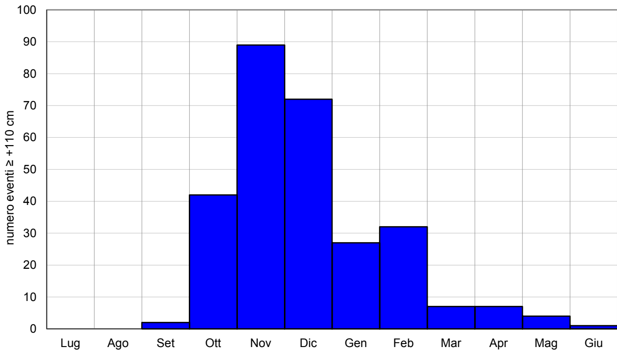
Figura 5 - Distribuzione mensile delle maree \geq +110 cm registrate a Venezia dal 1872 al 2015
