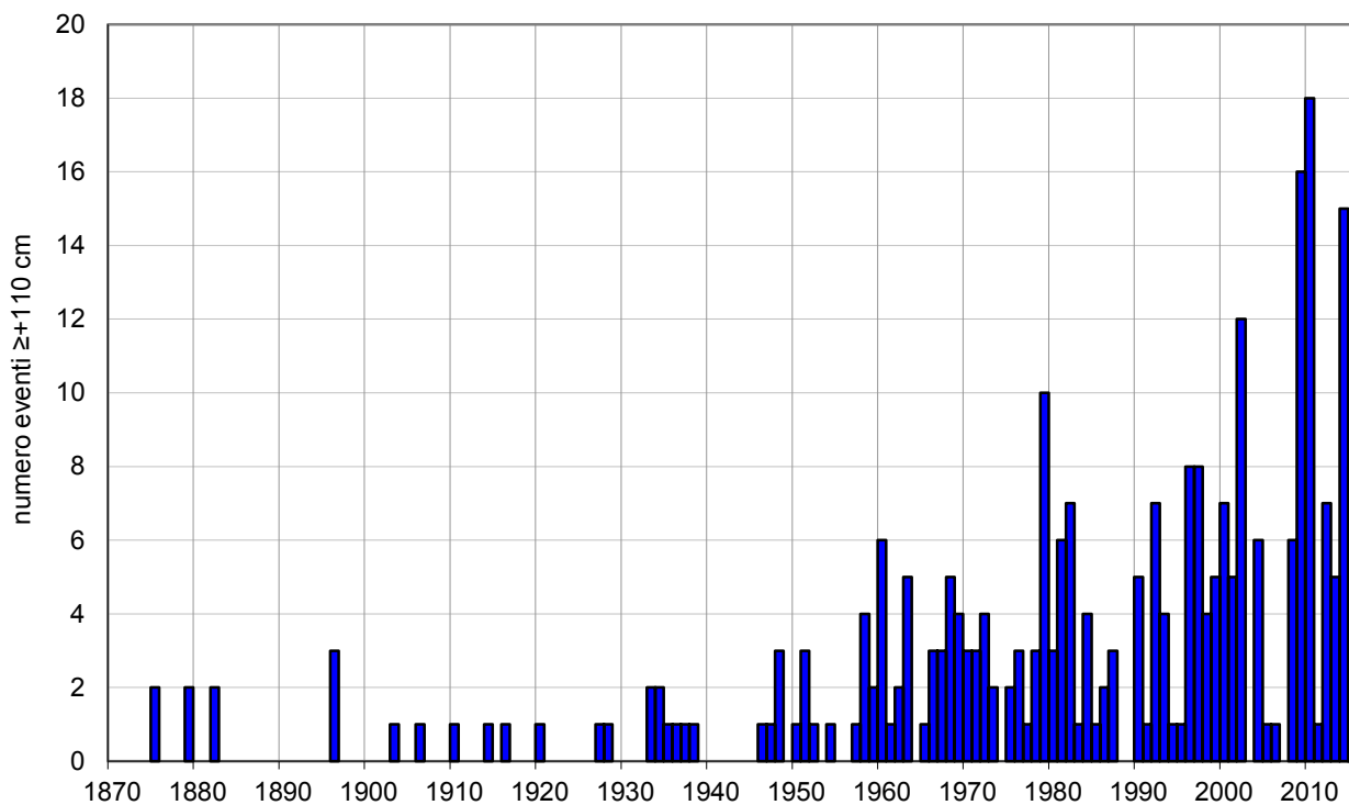
Figura 2 - Distribuzione annuale delle maree \geq +110 cm registrate a Venezia dal 1872 al 2015
